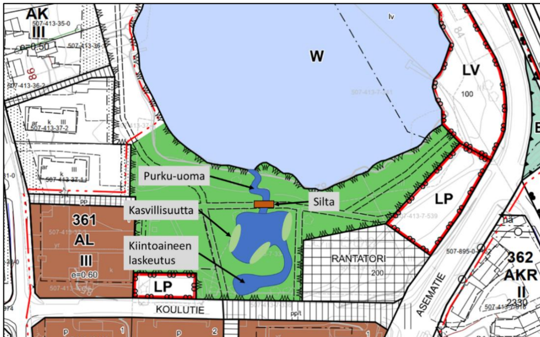
Kuva 19 Periaatepiirros hulevesialtaasta.
